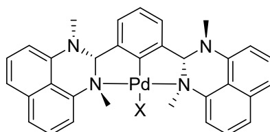
Figura 2.14 Compuesto tipo pinza N-C-N reportado por Chung.
