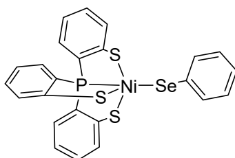
Figura 3.1 Diagrama de la molécula de Ni(III) con ligante fosfinotiolato de tres brazos.
