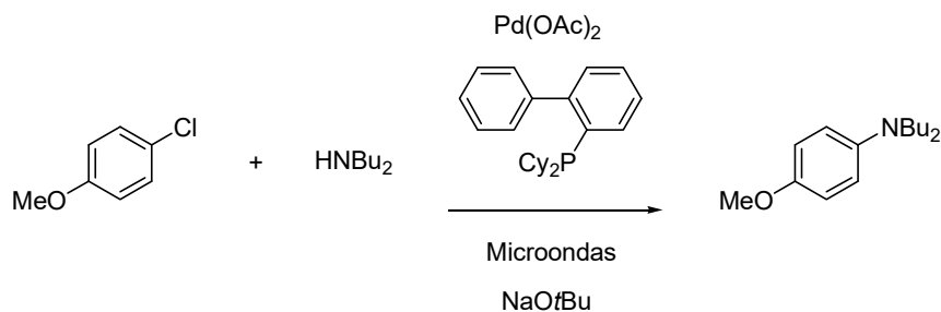
Figura 2.33 Sistema catalítico empleado para la aminación de clorobenceno asistida por microondas.
