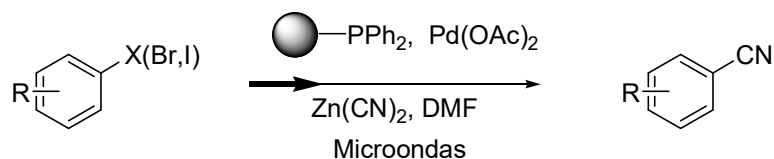
Figura 2.27 Cianación de halogenuros de arilo catalizada por paladio soportado.
