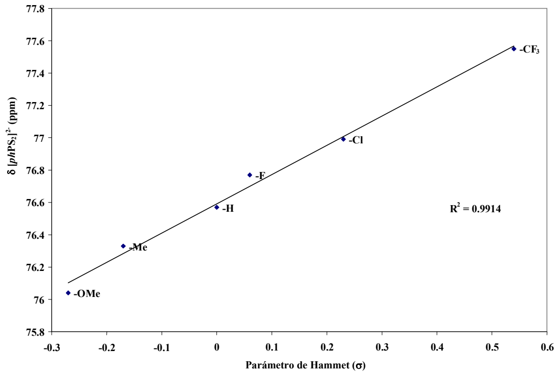
Figura 4.7 Desplazamiento químico ( \delta ) del fragmento [phPS_2]^{2-} vs. parámetro de Hammet ( \sigma ).
