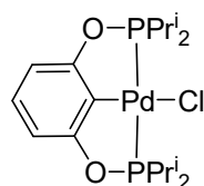
Figura 2.11 Compuesto fosfinito tipo pinza P-C-P.
