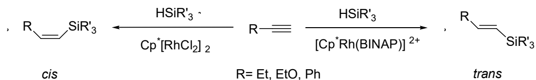
Figura 4.12 Selectividad para compuestos de rodio neutros y dicatiónicos.
