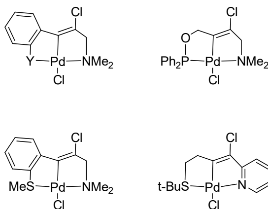
Figura 6. Esquema general de compuestos tipo pinza tipo Y-C-N.
