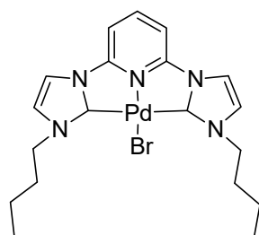
Figura 2.12 Diagrama del compuesto biscarbeneo tipo pinza C-N-C.
