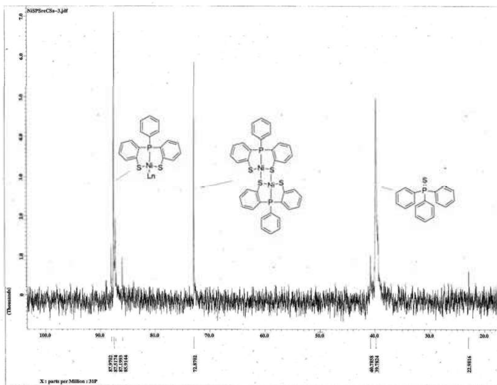
Figura 3.14 Espectro de RMN ^{31}\text{P}\{^1\text{H}\} (121 MHz, \text{CDCl}_3 ) a 25 °C de la mezcla de reacción de ariltiolación.
