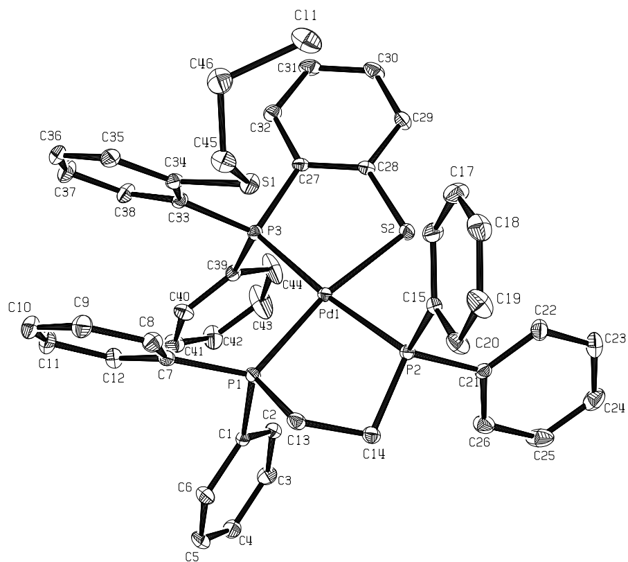
Figura 5.8 Una representación ORTEP de la estructura del catión \{[\text{Pd}[\text{phP}(\text{C}_6\text{H}_4\text{-}2\text{-SCH}_2\text{CH}_2\text{Cl})(\text{C}_6\text{H}_4\text{-}2\text{-S})] (\text{ph}_2\text{PCH}_2\text{CH}_2\text{Pph}_2)]\}^+ ( 20 ) a 50% de probabilidad.
