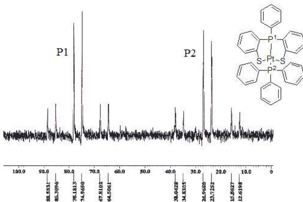
Figura 4.6 Espectro de RMN de ^{31}\text{P}\{^1\text{H}\} (121 MHz, \text{CDCl}_3 ) a 25 °C del compuesto [\text{Pt}(\text{phPS}_2)(\text{PPh}_3)] .
