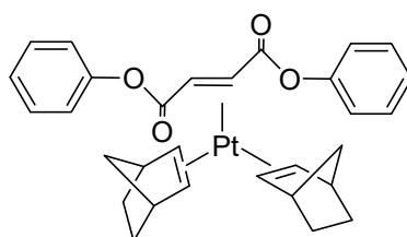
Figura 4.15 Esquema del compuesto empleado por Elsevier para la hidrosililación de estireno.
