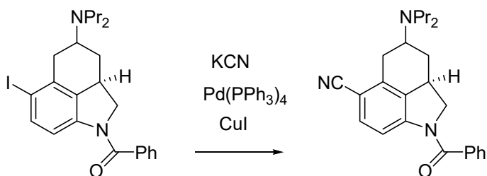
Figura 2.25 Esquema del compuesto en que Anderson lleva a cabo la cianación.
