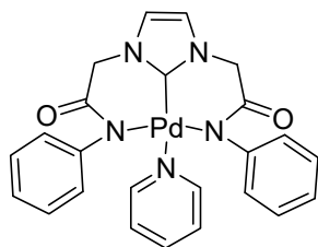
Figura 2.35 Diagrama del compuesto tipo pinza de Pd(II) N-C-N sintetizado por Lee. 45
