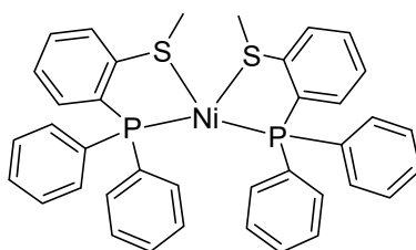
Figura 3.2 Compuesto de Ni(0) tetraédrico con ligantes fosfinotiolato.
