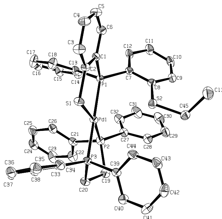
Figura 5.6 Una representación ORTEP de la estructura del catión \{[\text{Pd}[\text{phP}(\text{C}_6\text{H}_4\text{-2-SCH}_2\text{Cl})(\text{C}_6\text{H}_4\text{-2-S})](\text{ph}_2\text{PCH}_2\text{CH}_2\text{Pph}_2)]\}^+ ( 19 ) a 50% de probabilidad.
