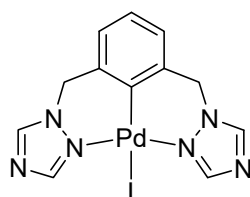
Figura 2.13 Compuesto tipo pinza N-C-N con 1,2,4-triazol.
