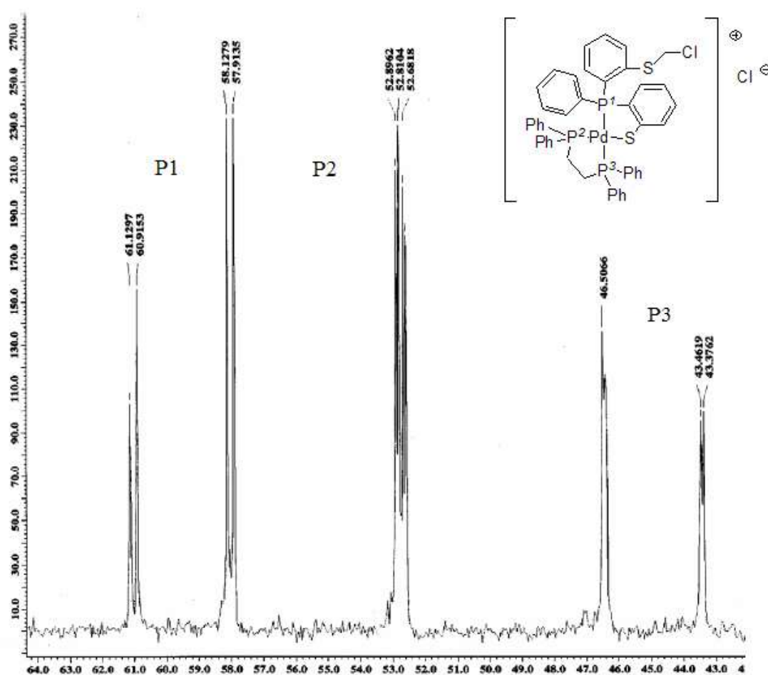
Figura 5.5 Espectro de RMN de ^{31}\text{P}\{^1\text{H}\} (121 MHz, \text{CDCl}_3 ) a 25 °C del complejo 19 .
