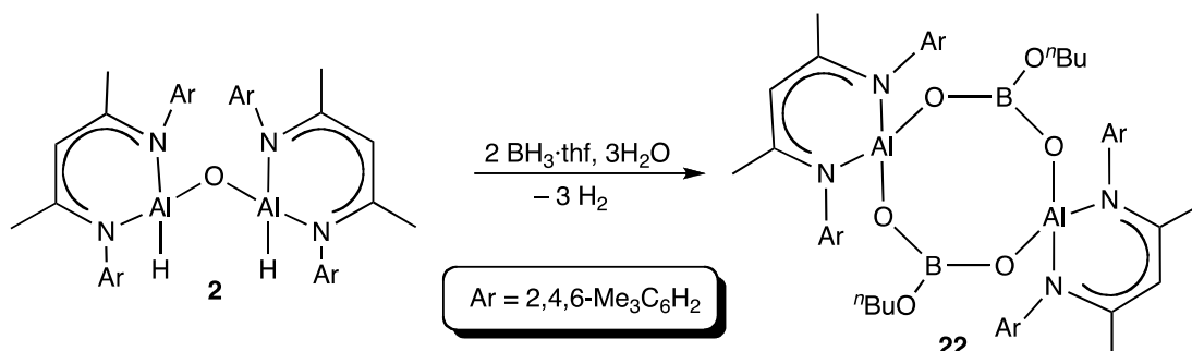
Esquema 5.10. Síntesis del alumoborato cíclico 22 .
