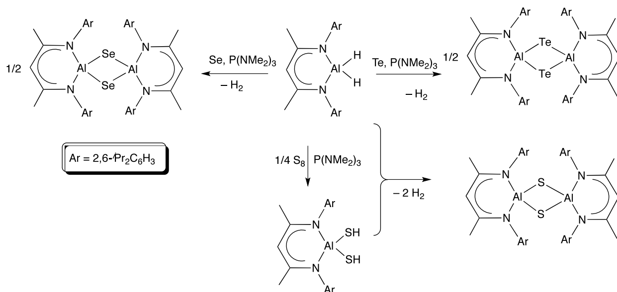
Esquema 2.1. Ruta de síntesis de los calcogenuros cíclicos [ iPr_LAl(\mu-E)_2Al^{iPr_L} ] ( E = S, Se, Te ; iPr_L = HC\{C(Me)N(Ar)\}_2 , ( Ar = 2,6\text{-}^iPr_2C_6H_3 )).
