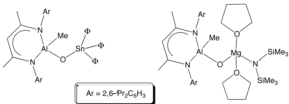
Figura 2.6. Compuestos heterobimetálicos Al-O-M conteniendo elementos representativos.
