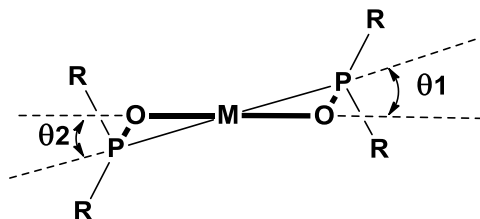
Esquema 57. Ángulos de torsión \theta .
