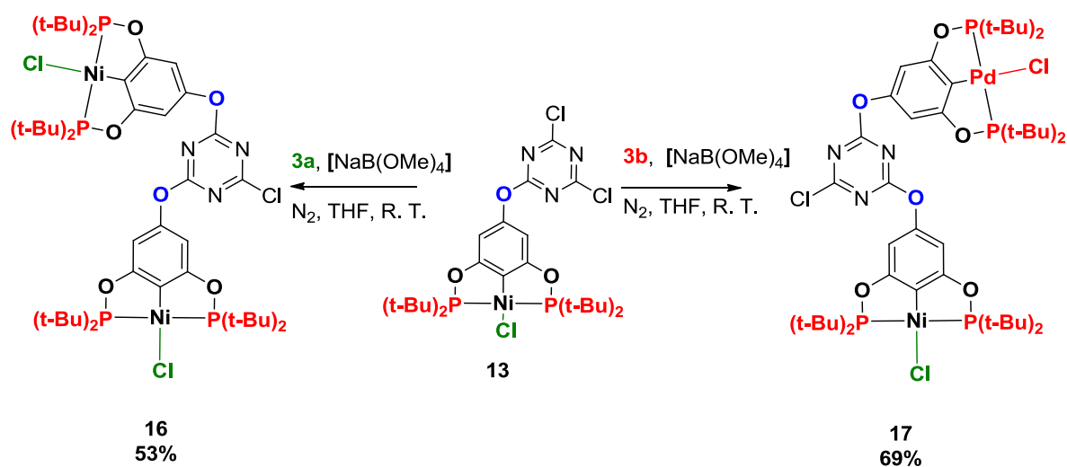
Esquema 42. Síntesis de éteres homo y heterodimetálicos a través de la adición de un segundo compuesto tipo pinza POCOP para -hidroxisusituidos.
